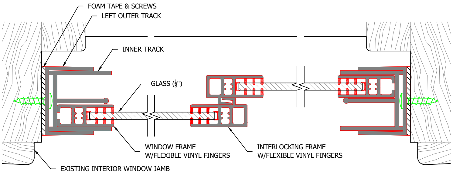
A - JAMB (FULL SCALE)
