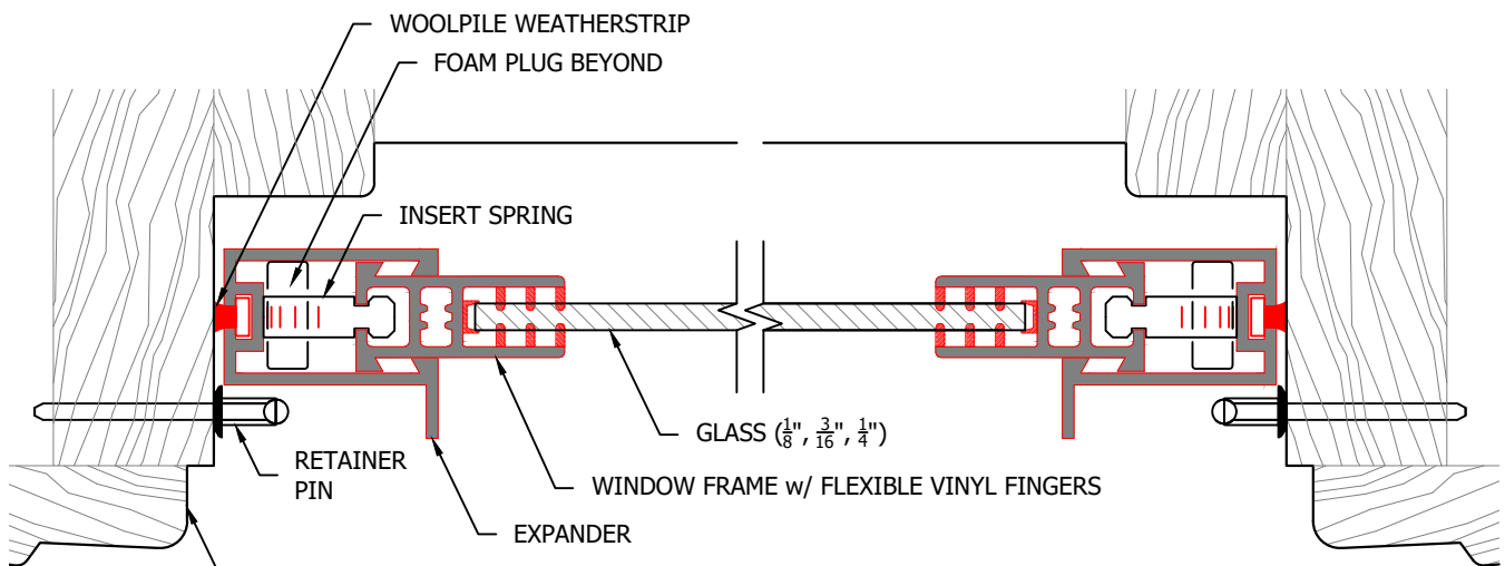
B - JAMB (FULL SCALE)
