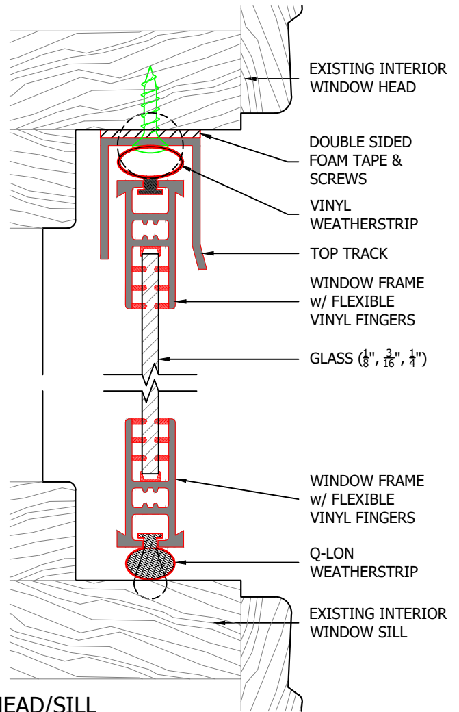
A - HEAD/SILL (FULL SCALE)
